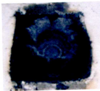
Рис.4. Внешний вид образцов после испытаний
