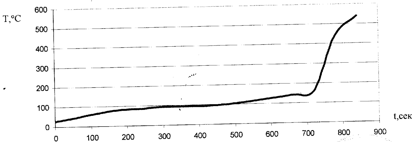
Рис. 8. Изменение температуры стальной основы образца с установленной на расстоянии 28 мм Плитой «Эндотерм 210104» толщиной 20 мм.
